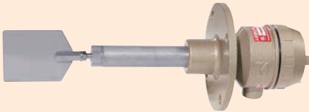
保護管延長式 NNL-8BS (安息角が大きい、タンク壁への付着が大きい場合等に、垂直取付・水平取付・斜め取付も可能)
