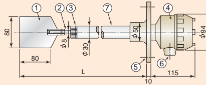
耐熱式 NNL-8BH (使用可能タンク内温度: 250℃以下)
