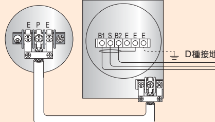
結線図
