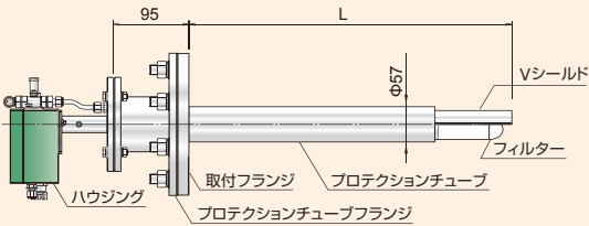
OXITEC 5000 (KEX-132□用)
