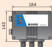
リークアラート73 (一体型)
