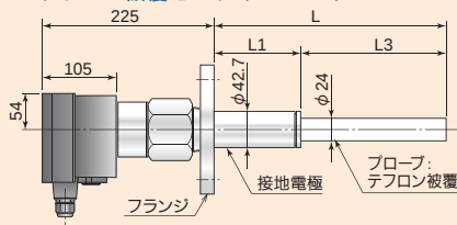
テフロン被覆センサ (～250℃)
