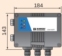
リークアラート65-02 (分離型)
