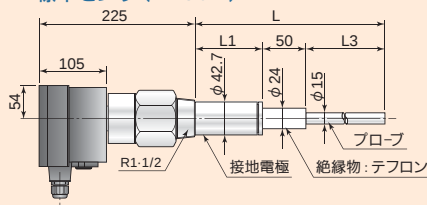
耐熱センサ (～400℃)
