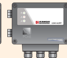
電源 4-20mA 出力 アラーム出力 1a x 2 (アラーム出力時と電源OFF 時 NO-COM 開)
