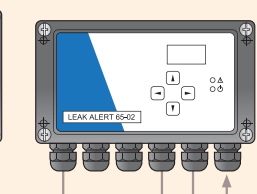
電源 4-20mA 出力 アラーム出力 1c 専用ケーブル max500m
