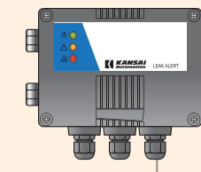
電源 4-20mA 出力 アラーム出力 1c 専用ケーブル max500m
