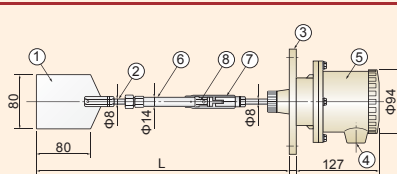
L寸法表 (8BA 軸長調整寸法)
