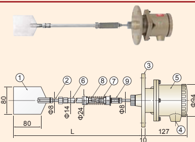
L寸法表 (8BA 軸長調整寸法)
