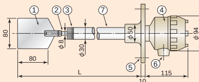
NL-8BS (保護管延長式)
