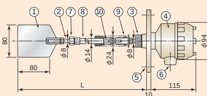
NL-8BA (振れ止めスプリング型)
