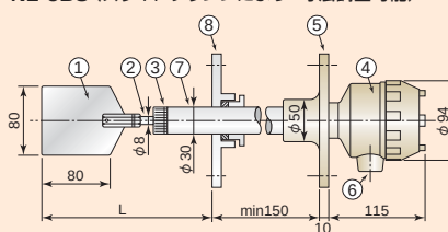
NL-8BS (スライドフランジによりL寸法調整可能)
