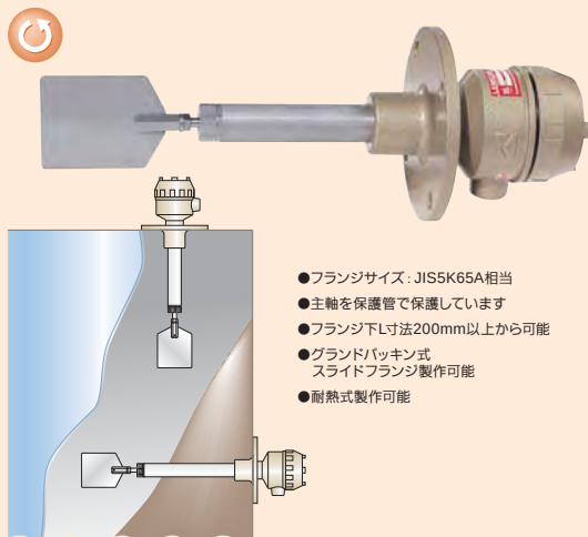
NL-8BS (保護管延長式)
