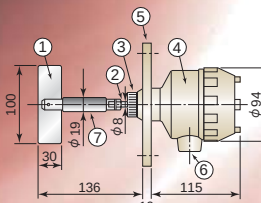
NL-8BF (フレキシブルシャフト)
