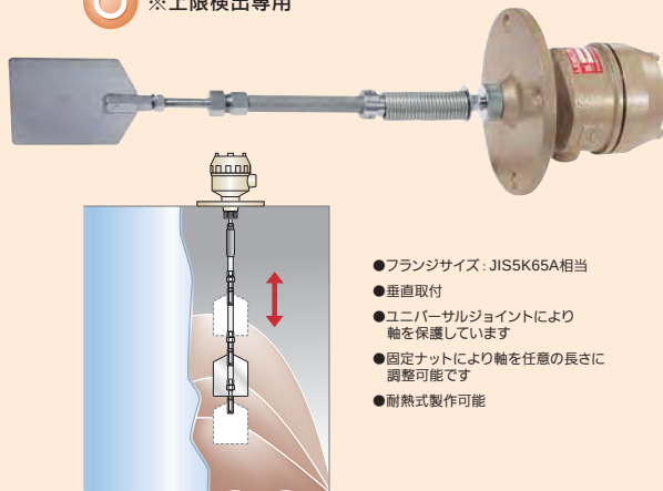
NL-8BA (振れ止めラバー型)
