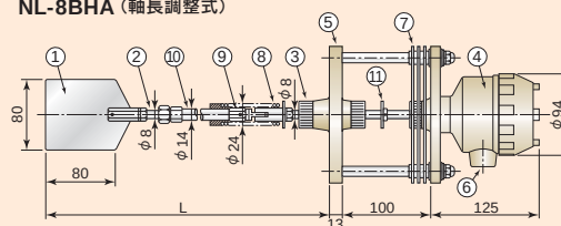
NL-8BHA (軸長調整式)
